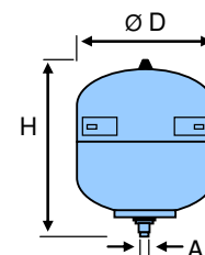
33-40 litrów z konsolą mocującą (widok z tyłu)
